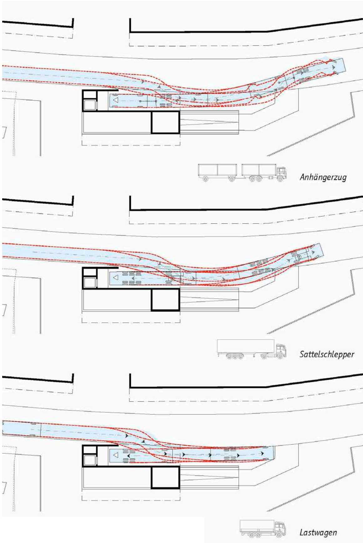
Anlieferung Coop Nutzfahrzeuge
