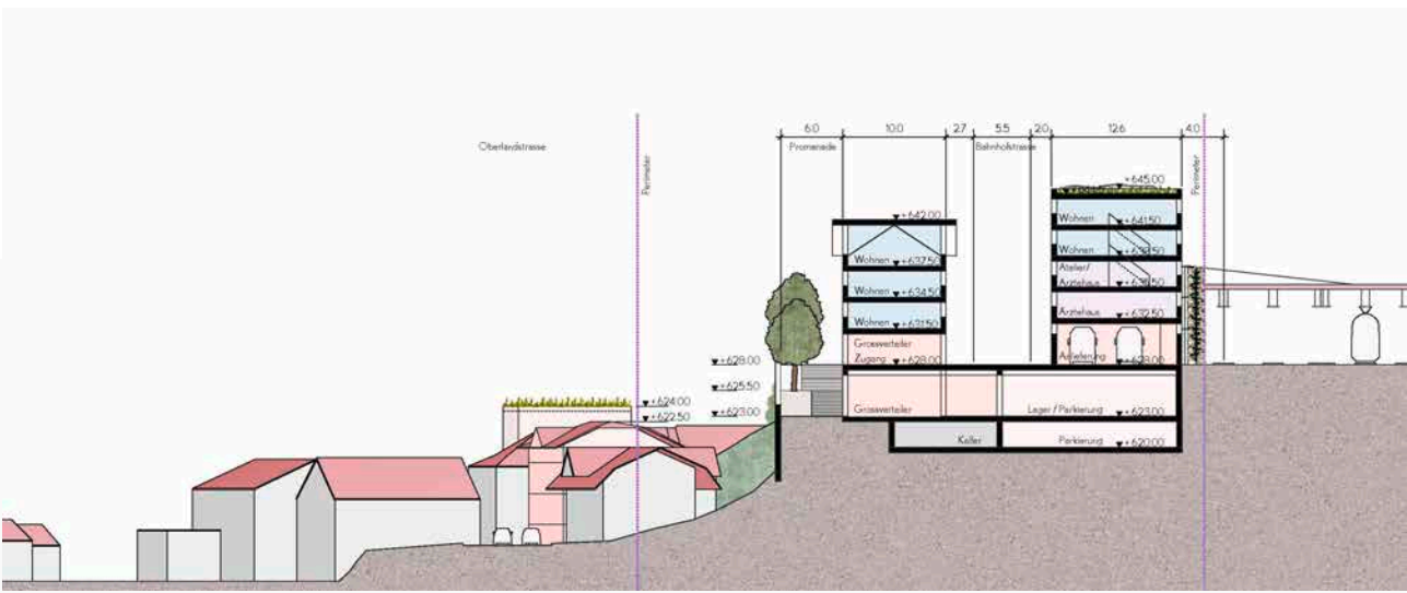
Schnitt B – B
