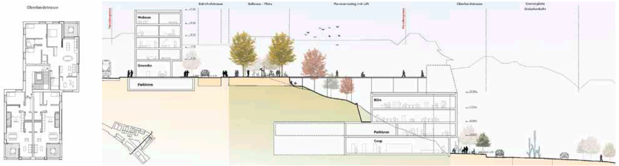
Regelgeschoss Wohnen | Querschnitt Coop
